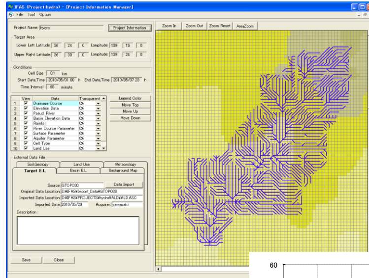
自動作成した落水線 表示例
