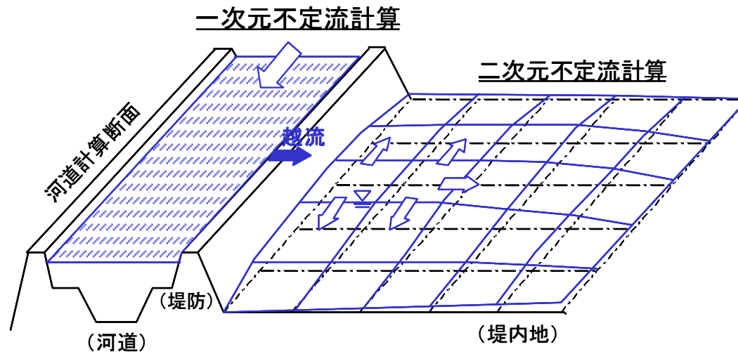
氾濫解析モデルの概要
