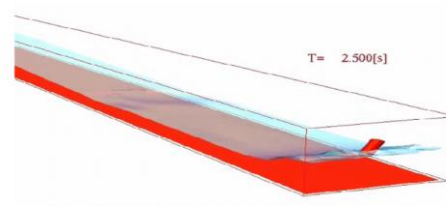
防波堤越流挙動
