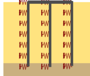
杭バネのモデル
